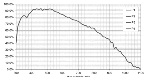
MV-CU060-60GM V2
