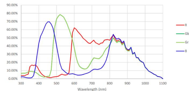
MV-CU060-60GC V2
